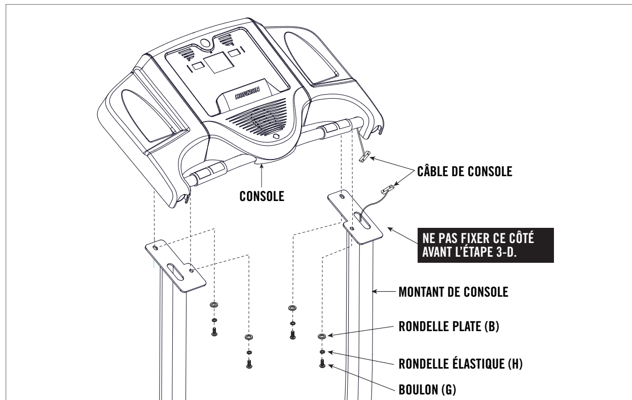
RONDELLE ÉLASTIQUE (H) 15 mm Quantité : 4
